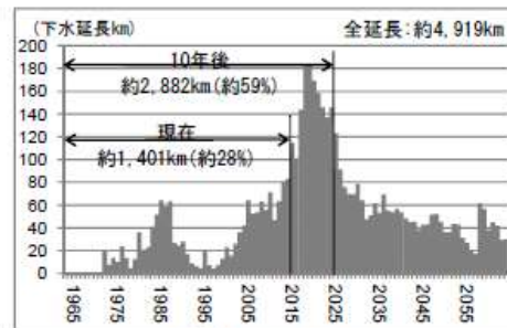
下水道(耐用年数:50年)
