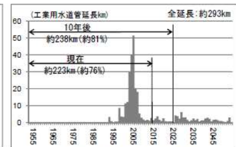
工業用水道管(耐用年数:40年)
