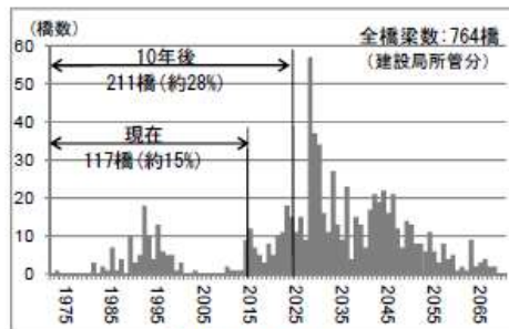
橋梁(耐用年数:60年)
