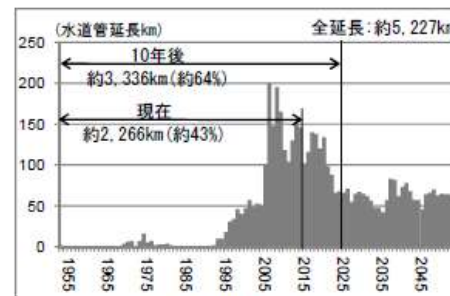
水道管(耐用年数:40年)
