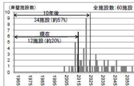
岸壁(耐用年数:50年)
